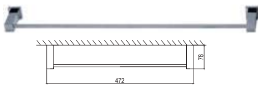
Toallero barra 40 cm de latón y zamak, cromo Towel bar 40 cm, brass and zamak, chrome Barre à serviette 45 cm en laiton et zamak, chrome Portasciugamani 45 cm, in ottone e zamak, cromato
